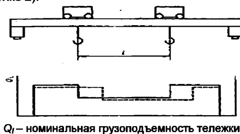
Рисунок 2 – Пример ограничения при оснащении крана двумя тележками
